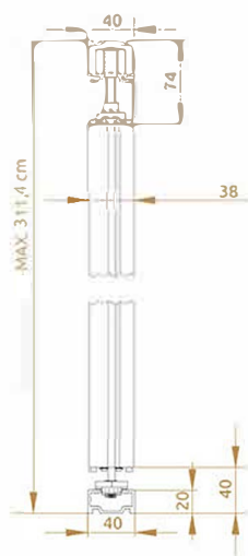
WIDOK Z PRZODU - LAMELA
