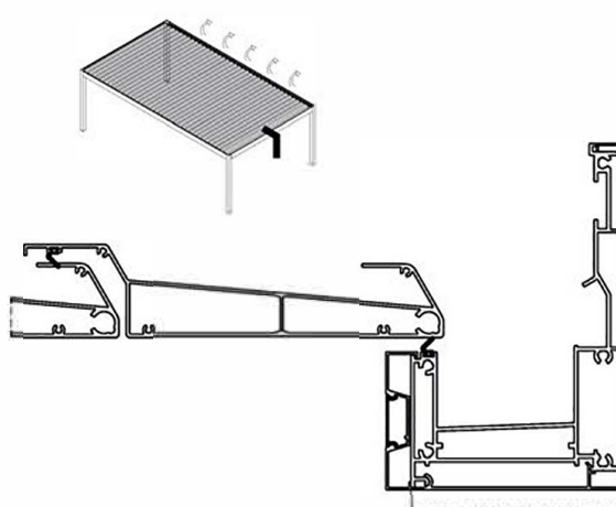
Przekrój prowadnicy poprzecznej
