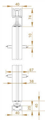
WIDOK Z PRZODU - LAMELA
