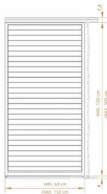
WIDOK Z PRZODU - LAMELA
