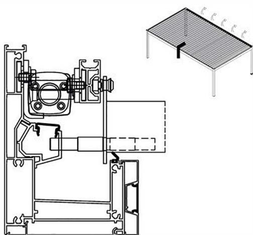
Przekrój prowadnicy podłużnej
